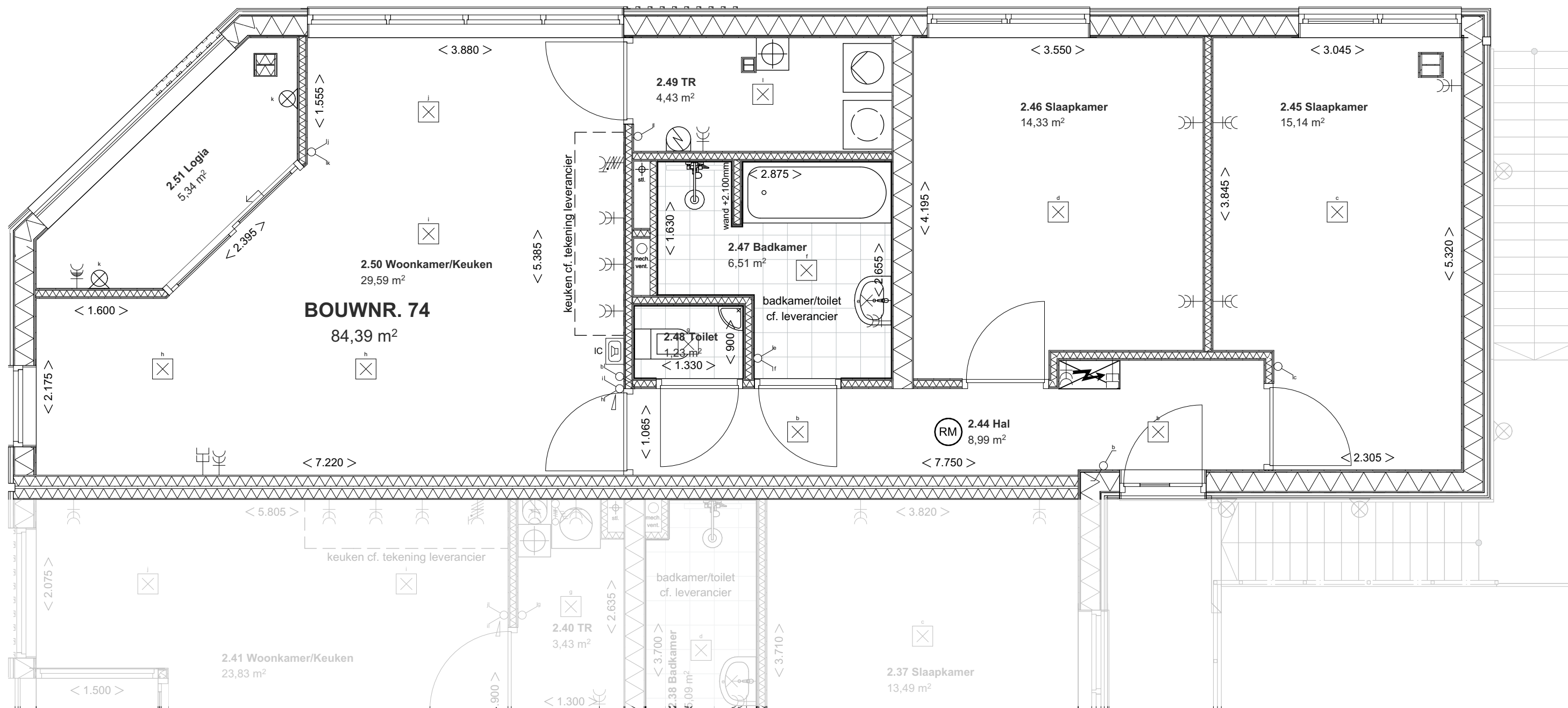
PLATTEGROND - 1:50
