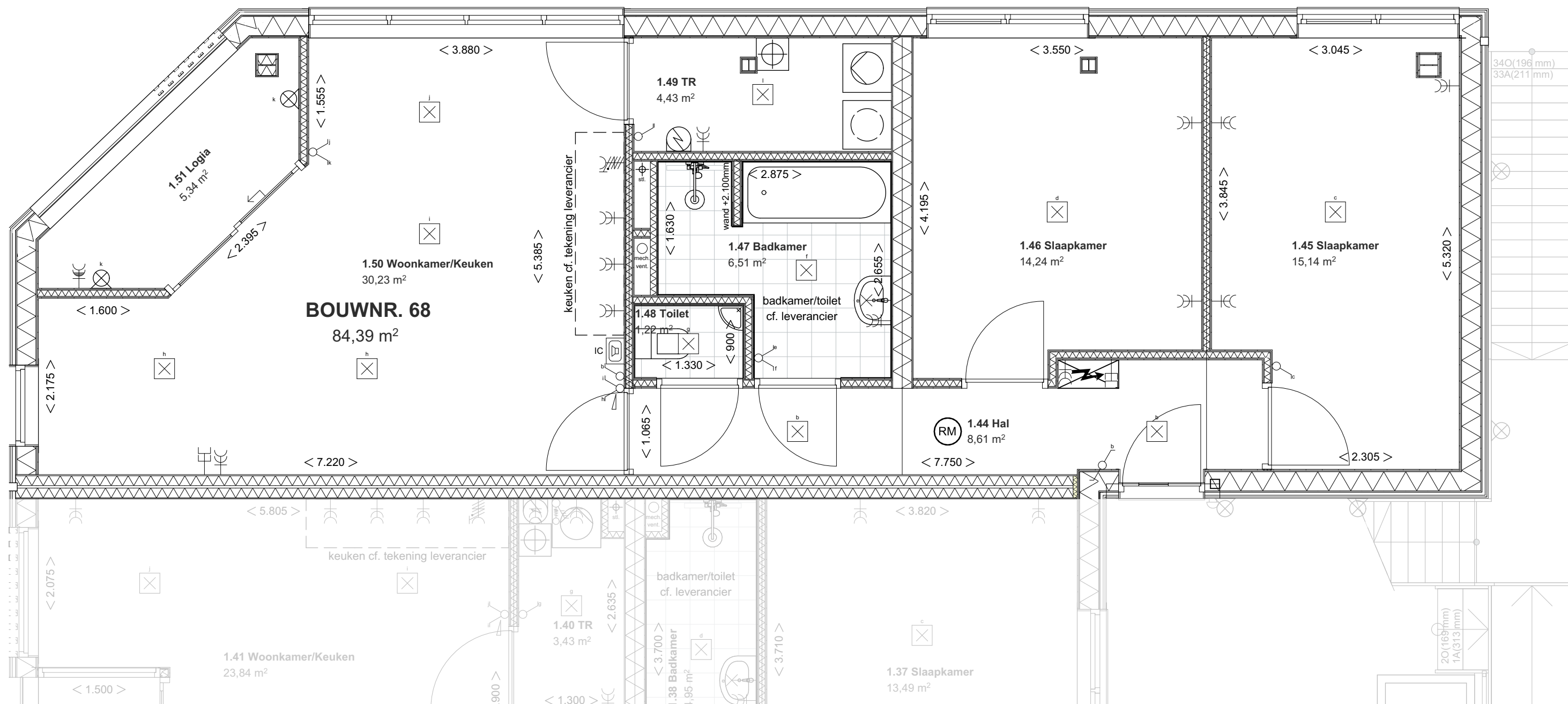
PLATTEGROND - 1:50
